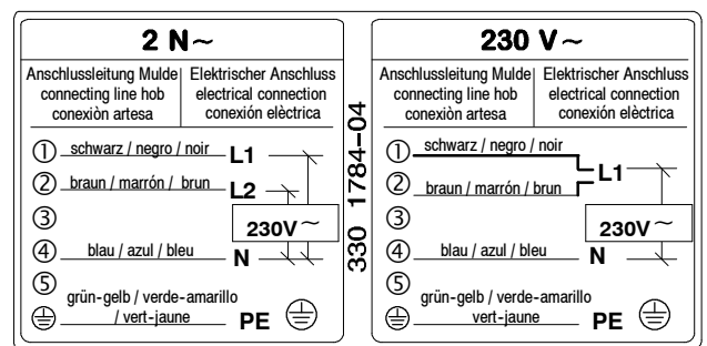
Anschluss-Schema 230 V ~
