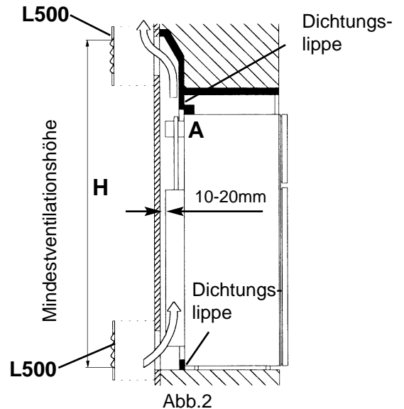
Installation mit oberem und unterem Lüftungsgitter (L500).
