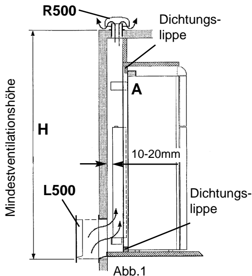
Installation mit Dachentlüfter (R500) und unterem Lüftungsgitter (L500).
