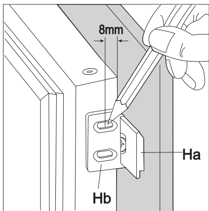
Abb. 18: Tür des Gerätes und die des Möbels um ca. 90° öffnen. Winkelstücke (Hb) auf die Türmitnehmer setzen (Ha). Geräte- und Möbeltür aneinander halten und die Löcher an der Gerätetür markieren.
