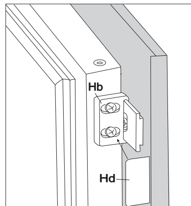
Abb. 21: Die Abdeckung (Hd) in das Winkelstück (Hb) eindrücken, bis sie einrastet.
