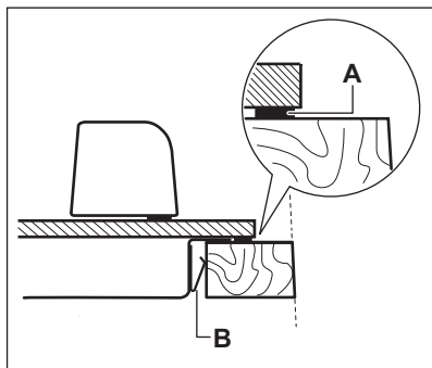
A) capa impermeabilizante B) abrazaderas montadas
