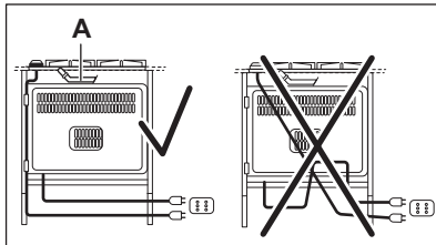
A) Condotta rigido in rame o tubo flessibile in acciaio inox
