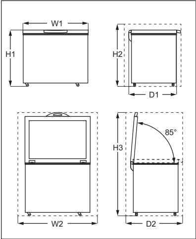
Dimensiones generales 1)
