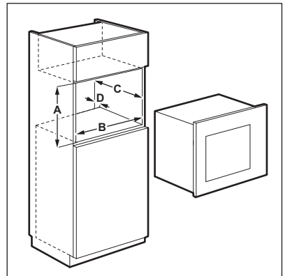
Distances d'installation
